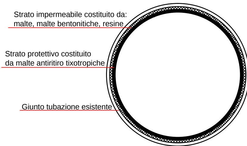
Sezione trasversale
