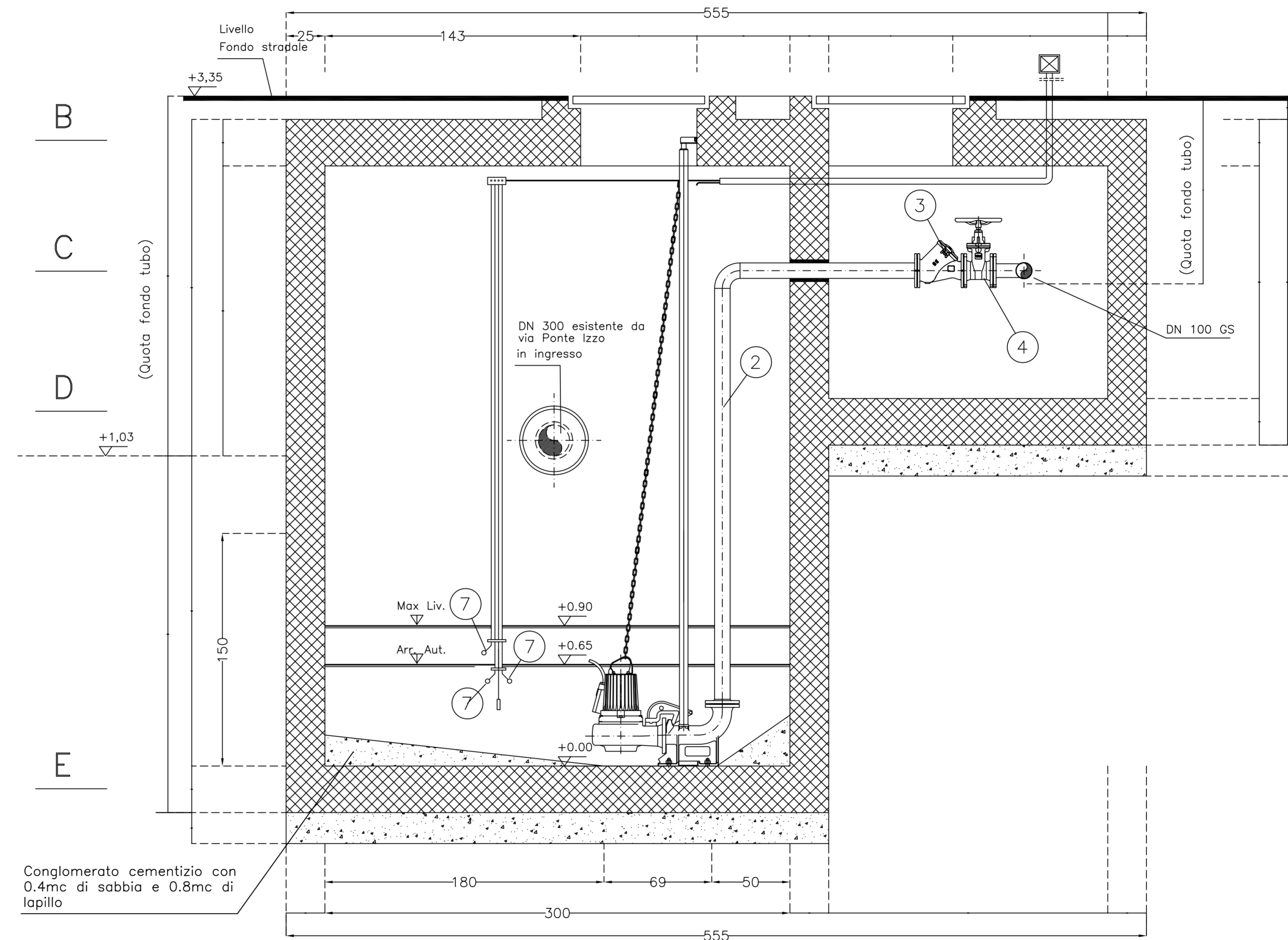
Sez. A-A' 1:20
