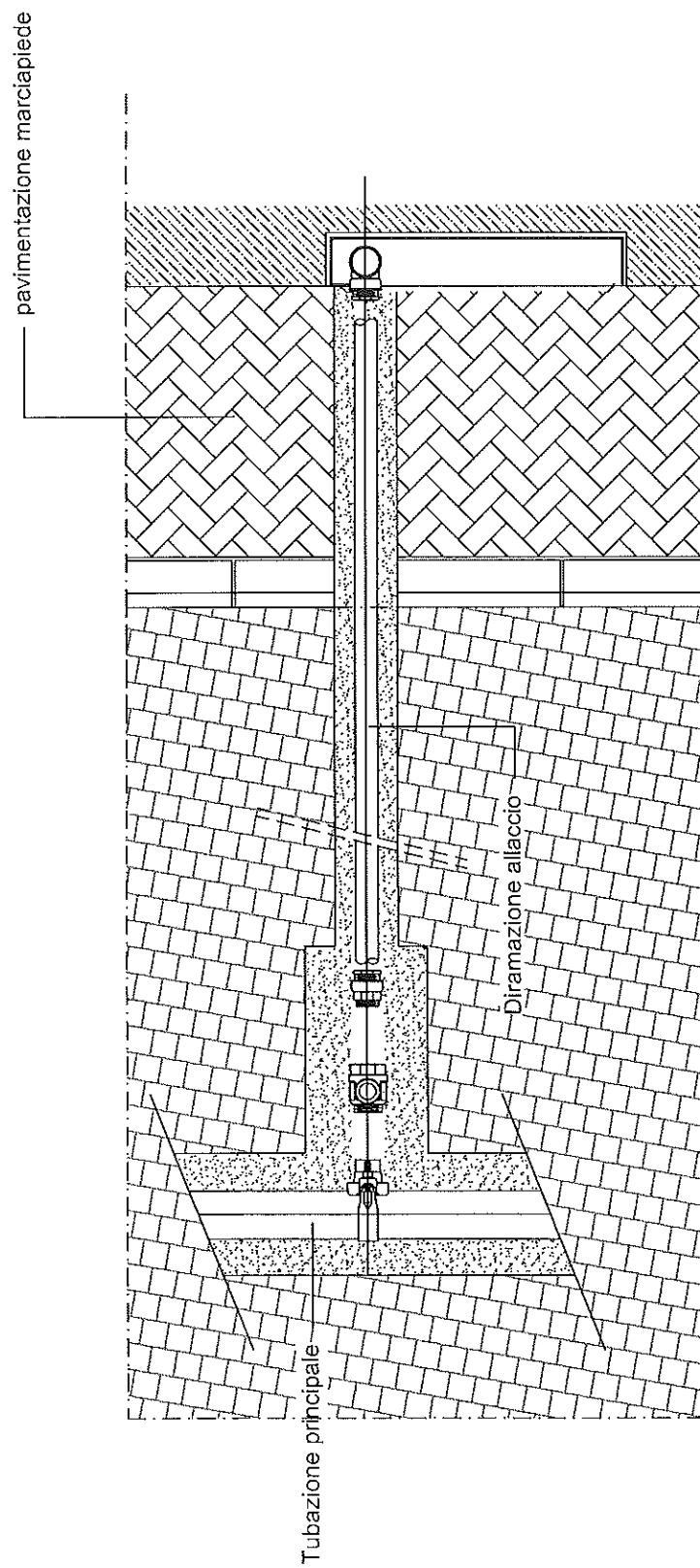
SCHEMA B3 Allaccio idrico - Pavimentazione in Cubetti
